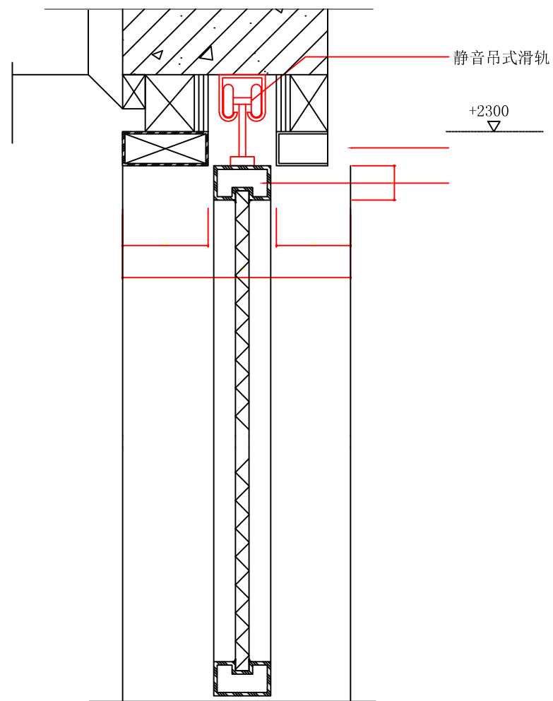
① DR1大样图 1:5
