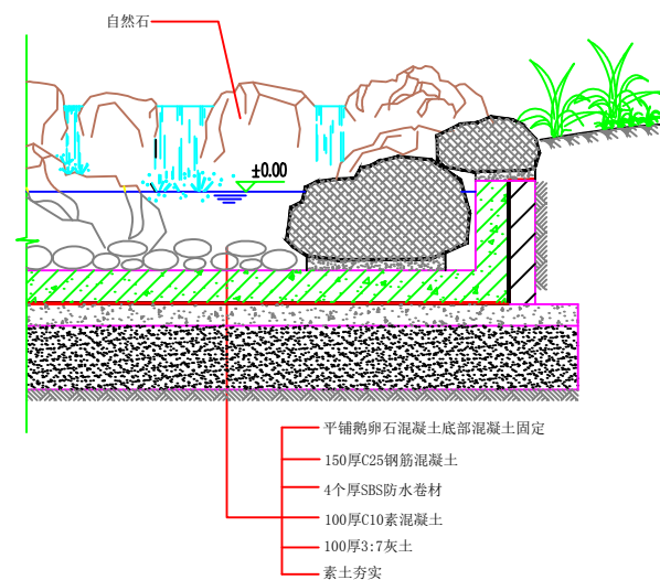
② 河道立断面图
