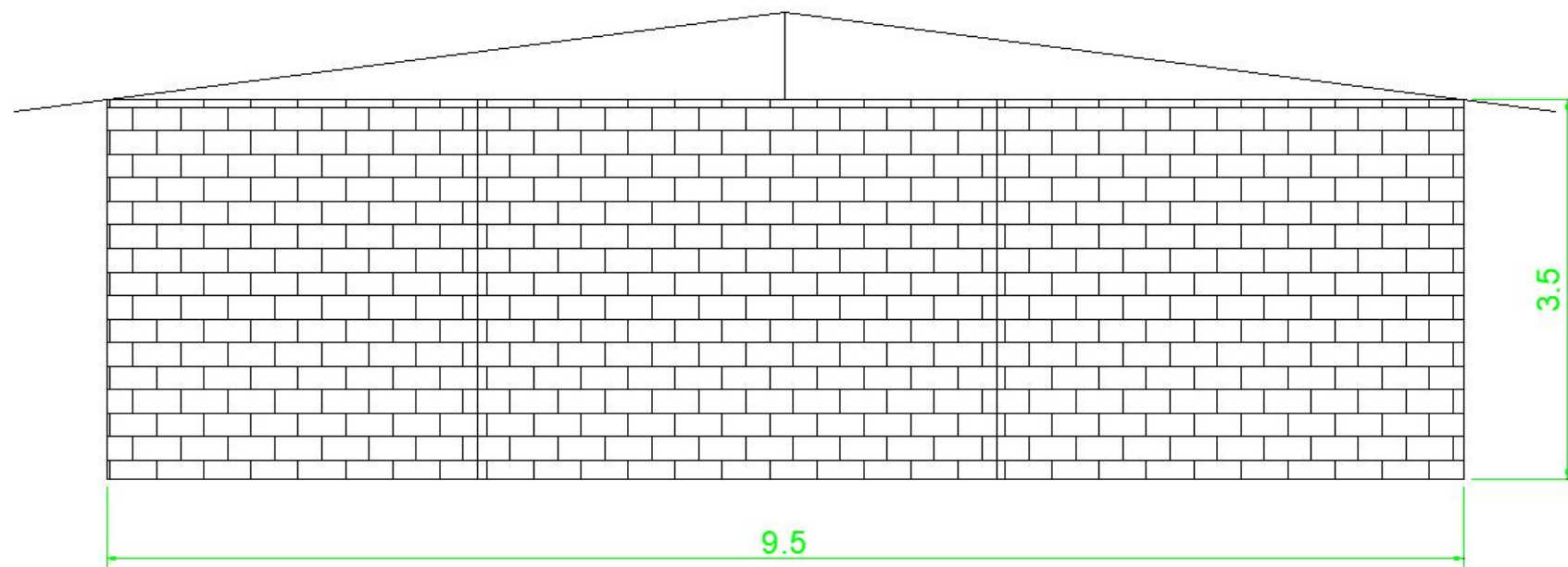
侧面图
