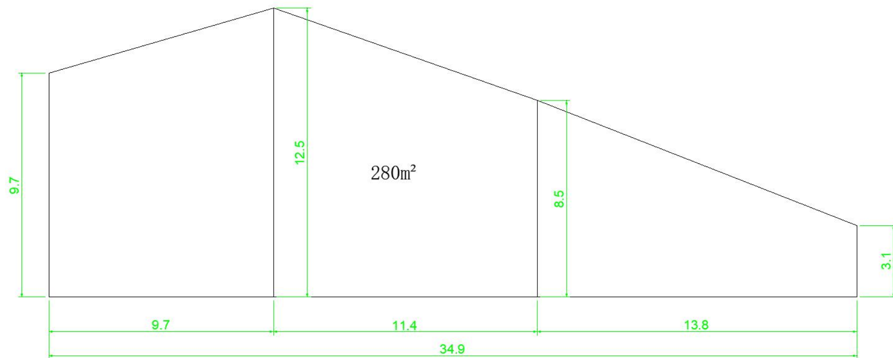
平面图
